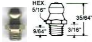
CODIGO: 0447 GRASERA # 100 MARCA INDUX USA
