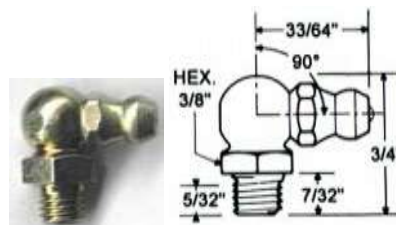
CODIGO: 0451 GRASERA # 190 MARCA INDUX USA
