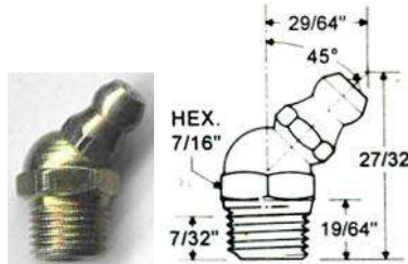
CODIGO: 0453 GRASERA # 245 MARCA INDUX USA
