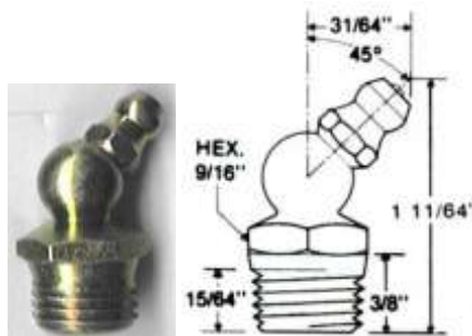
CODIGO: 0456 GRASERA # 345 MARCA INDUX USA
