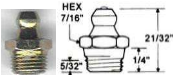
CODIGO: 0452 GRASERA # 200 MARCA INDUX USA
