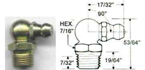
CODIGO: 0454 GRASERA # 290 MARCA INDUX USA
