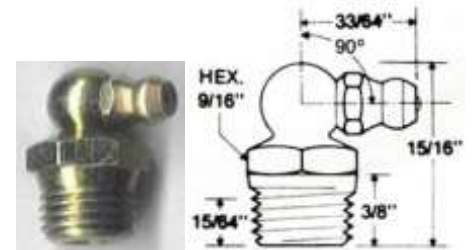
CODIGO: 0457 GRASERA # 390 MARCA INDUX USA
