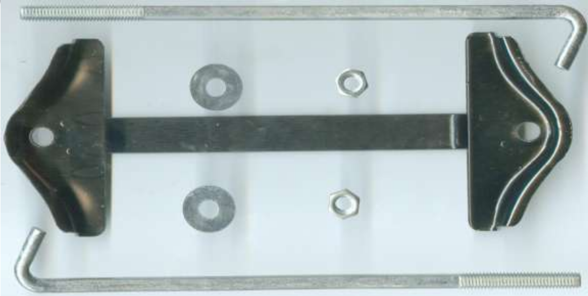
CODIGO: 0789 SOPORTE ACUMULADOR AMERICANO JUEGO DE 7 PIEZAS
