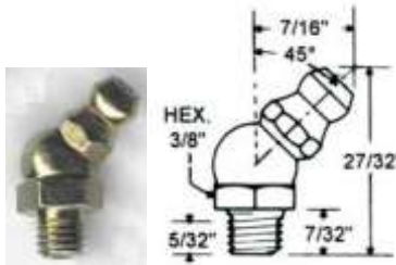
CODIGO: 0450 GRASERA # 145 MARCA INDUX USA
