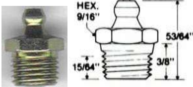
CODIGO: 0455 GRASERA # 300 MARCA INDUX USA
